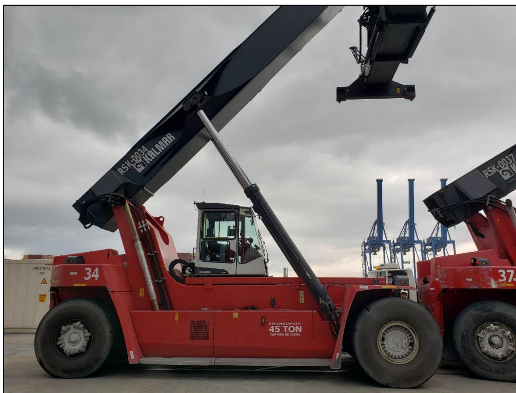
Figura 1. Empilhadeira de grande porte (Reach-Stacker), RSK-0034.
