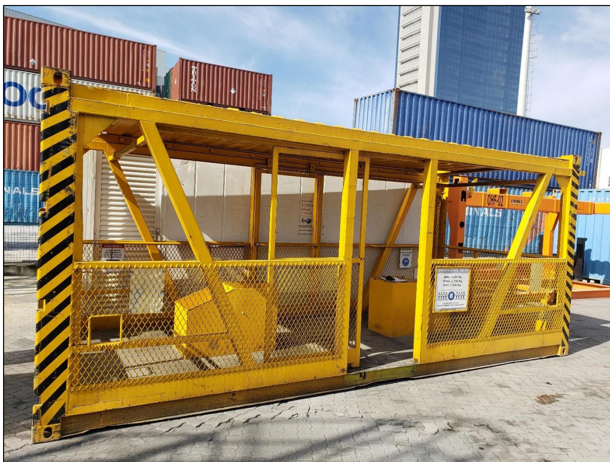
Figura 1. Safty Cage - 02
