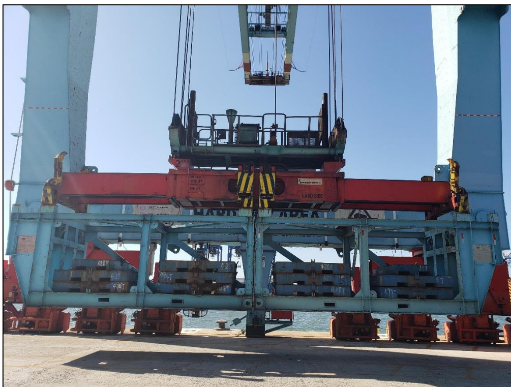
Figura 5. Teste de carga – Twin Lift.
